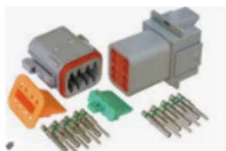
Deutsch plug 8 pin kit – ETDP8P
